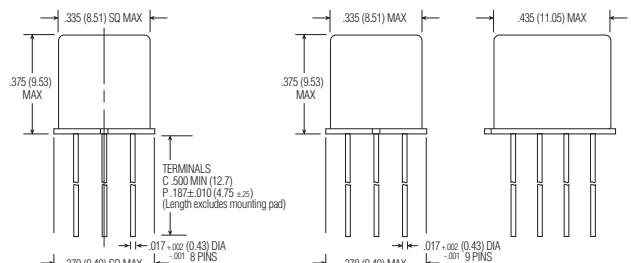
MGS/MGSD/MGSDD ENCLOSURE
