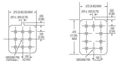
MGS/MGSD/MGSDD HEADER
