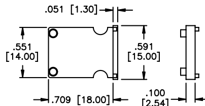
PICODA2 Spacer
