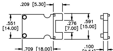
PICODAH2 Spacer
