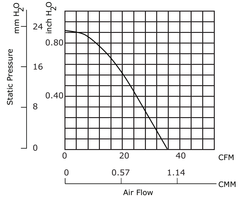
CBM-A232B-125
