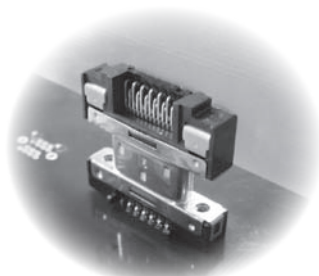
Vertical connection type 垂平连接式
