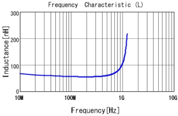
LQG15HN56NJ02 L
