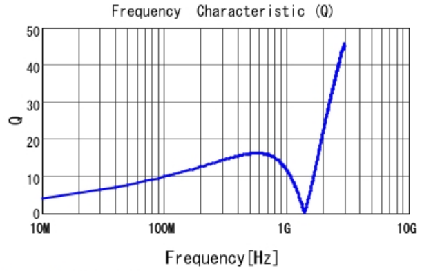
LQG15HN56NJ02 Q
