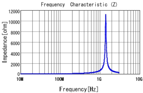
LQG15HN56NJ02 |Z|
